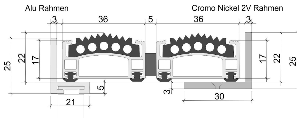
Schwerlastprofil - Gummi Höhe 22mm
